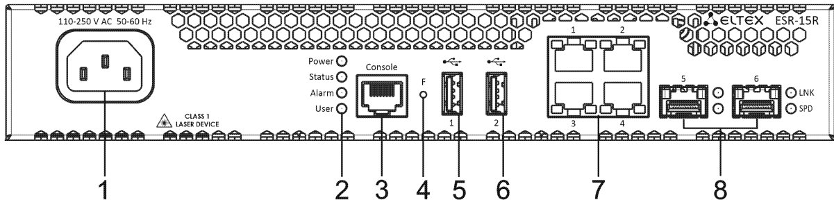
Рисунок 40 – Передняя панель ESR-15R
