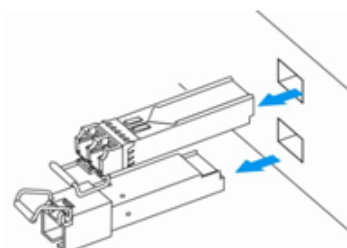
Рисунок 65 – Извлечение SFP-трансиверов
