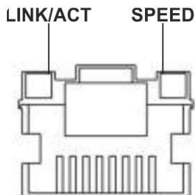
Рисунок 51 – Расположение индикаторов разъема RJ-45
