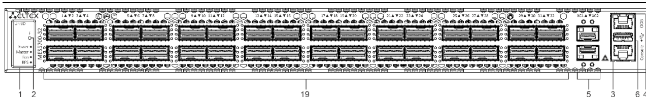
Рисунок 36 – Передняя панель MES5700-32
