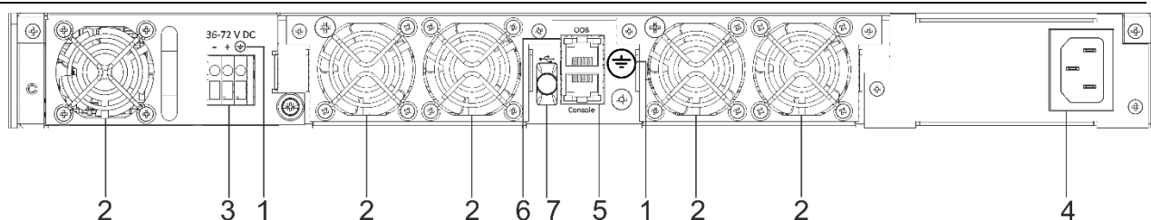
Рисунок 63 – Задняя панель MES5400-48
