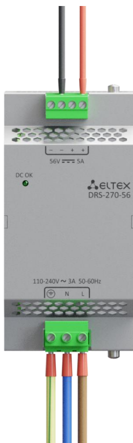
Рисунок 106 – Подключение питания к DRS-270-56
