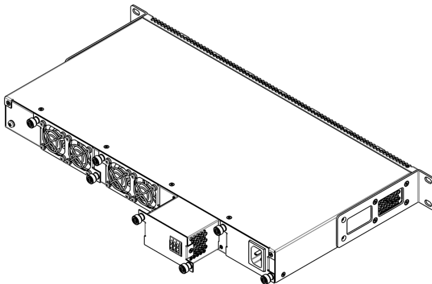
Рисунок 109 – Установка модулей питания
