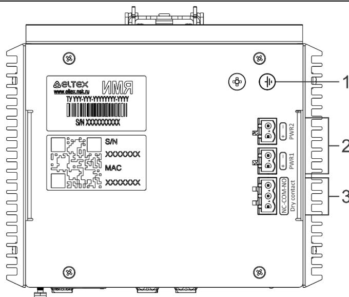
Рисунок 41 – Верхняя панель MES3500I-8P8F
