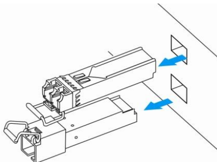
Рисунок 113 – Извлечение SFP-трансиверов
