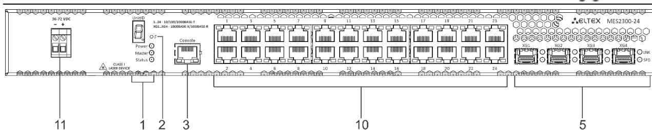
Рисунок 4 – Передняя панель MES2300-24 DC
