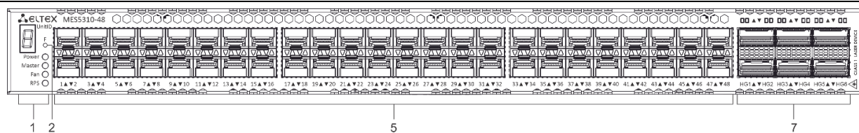
Рисунок 30 – Передняя панель MES5310-48
