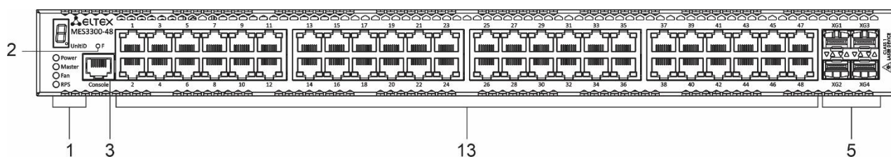
Рисунок 20 – Передняя панель MES3300-48
