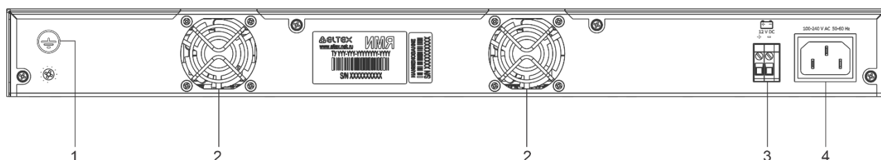
Рисунок 50 – Задняя панель MES2300B-48
