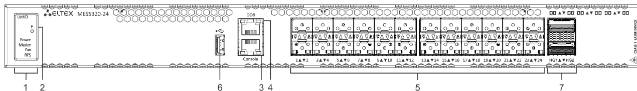
Рисунок 31 – Передняя панель MES5320-24
